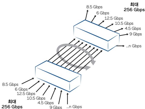
프레임 기반 트렁킹 IOD(In-Order Delivery)를 유지하는 ASIC
